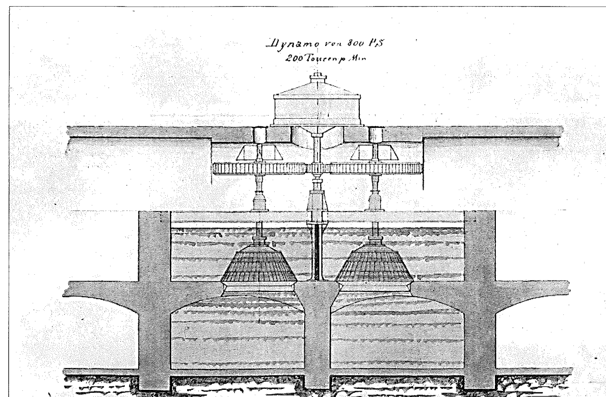
Vesivoimalaitoksen kuva edestäpäin, josta on nähtävissä kaksi vesiturbiinia ja yksi keskellä oleva generaattori.
