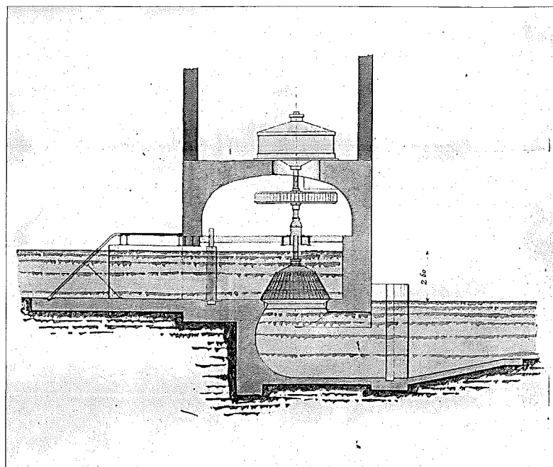
Kiviniemen koskeen suunnitellun vesivoimalaitoksen kaavakuva sivultapäin.
