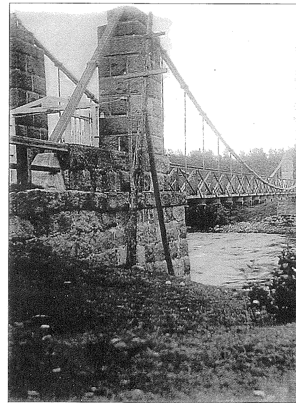
Kiviniemen ketjuriippusilta eri vinkkeleistä kuvattuna. Silta palveli tieliikennettä vuodet 1877-1939.
