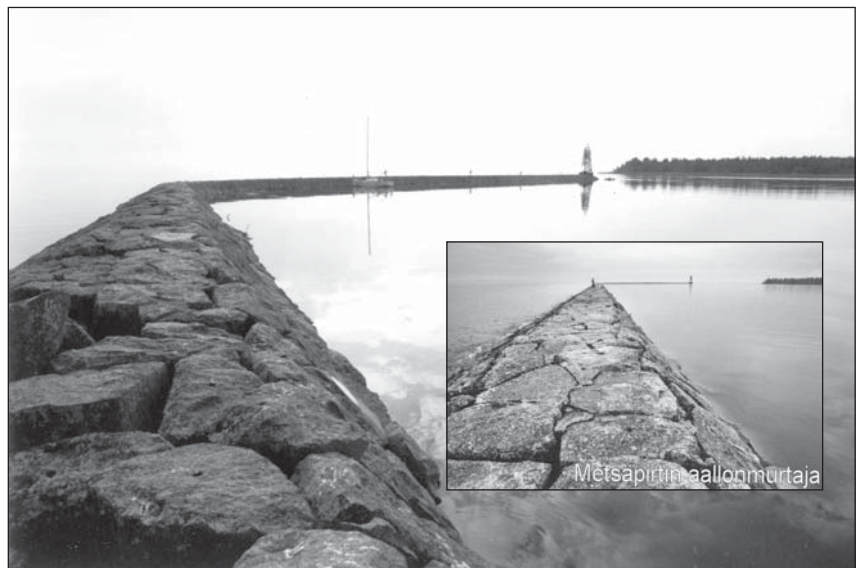
Saaroisten aallonmurtaja.
